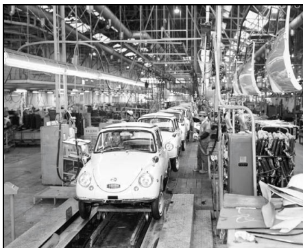
群馬製作所本工場 生産ライン(1961年)
